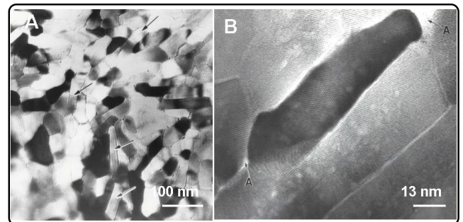
Figura 8. A) Imágenes de MET de los cristales que conforman los prismas del esmalte dental humano. B) A mayor amplificación. Nótese la presencia de la línea oscura (indicada por flechas en (A)) y la existencia de material orgánico rodeando los cristales de HAP (indicado por flechas con la letra "A").
