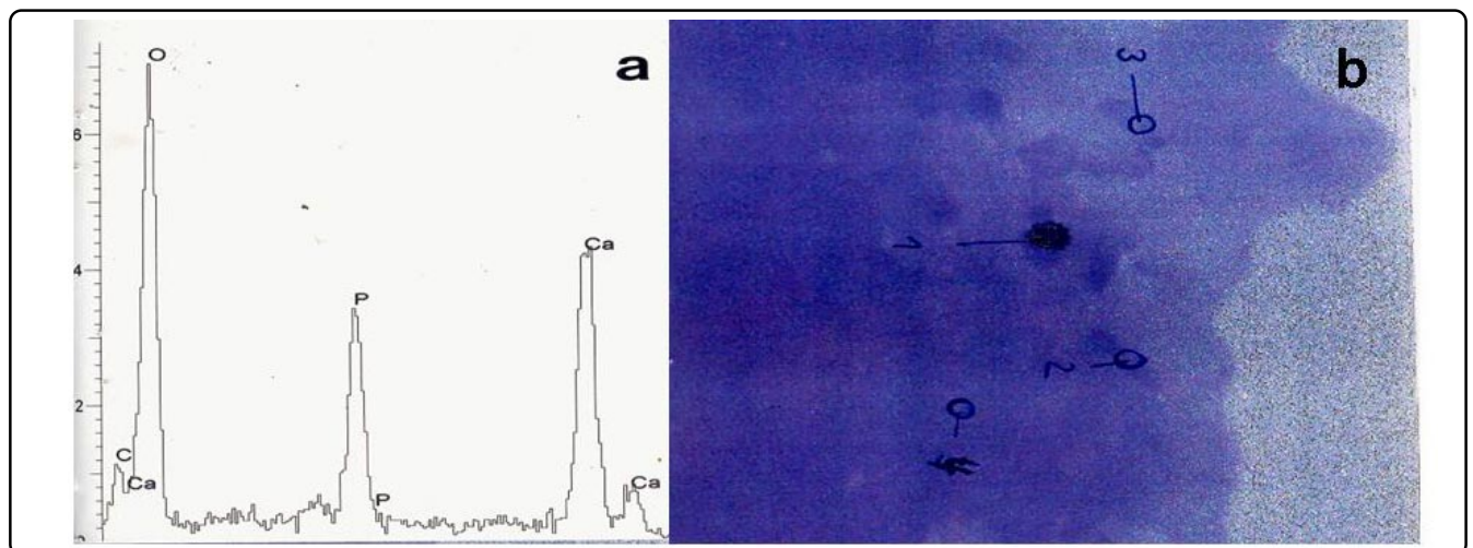
Figura 3. A) Espectro de rayos X característicos (EDS) del esmalte dental humano. Se observa la presencia de Ca, P y O. B) Imagen de MET del esmalte dental humano.
